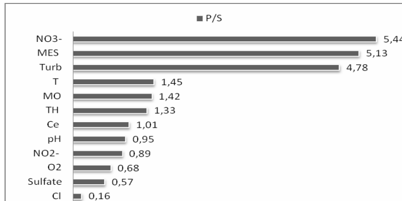
Figure 14:- Le rapport saisonnier (saison de pluie /saison sèche)
