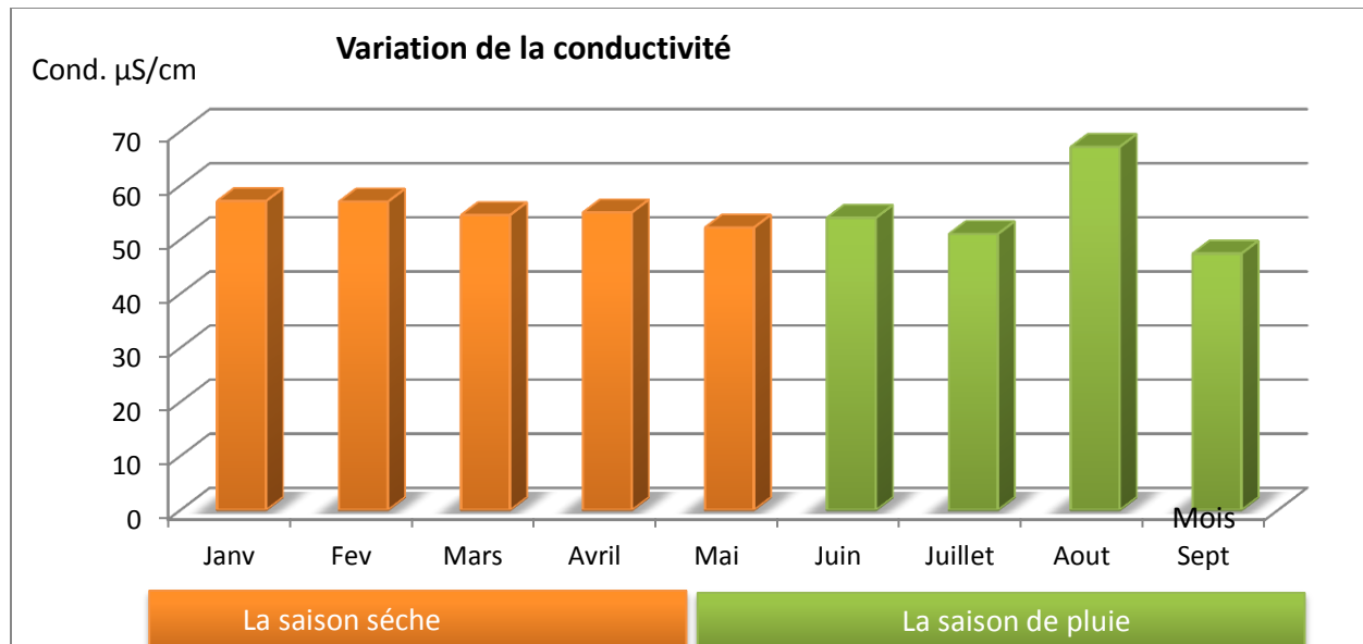
Figure 5:- Variation de la conductivité
