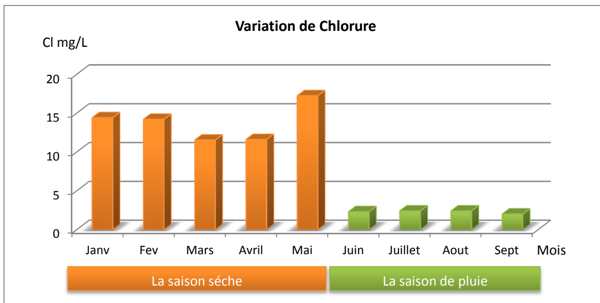
Figure 13:- Variation de Chlorure
