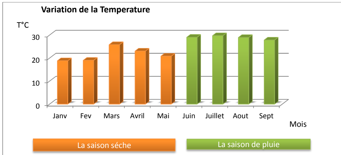
Figure 2:- Variation de la température
