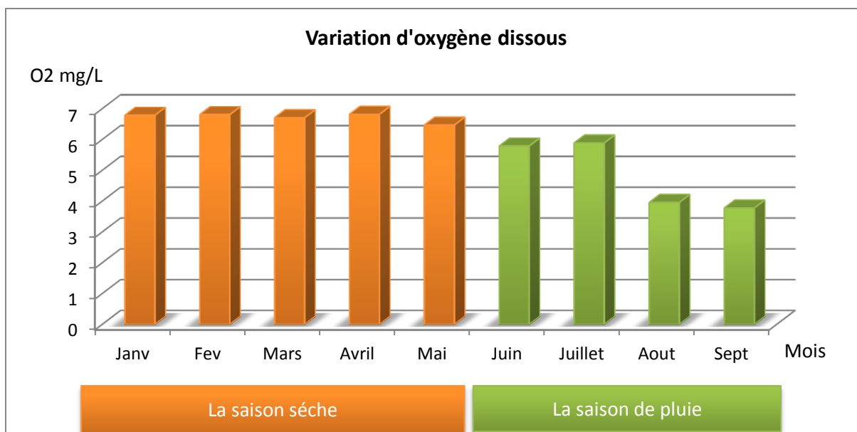
Figure 10:- Variation d'Oxygène dissous entre les saisons de l'année.
