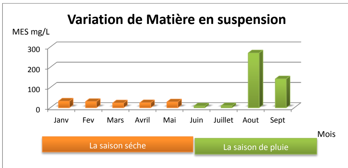
Figure 8:- Variation de la MES
