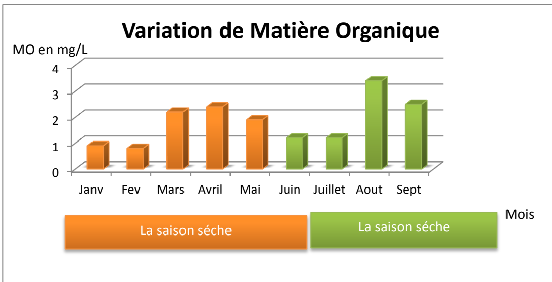
Figure 9 : Variation de la matière organique
