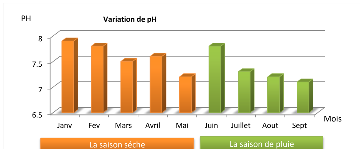
Figure 3:- Variation du pH
