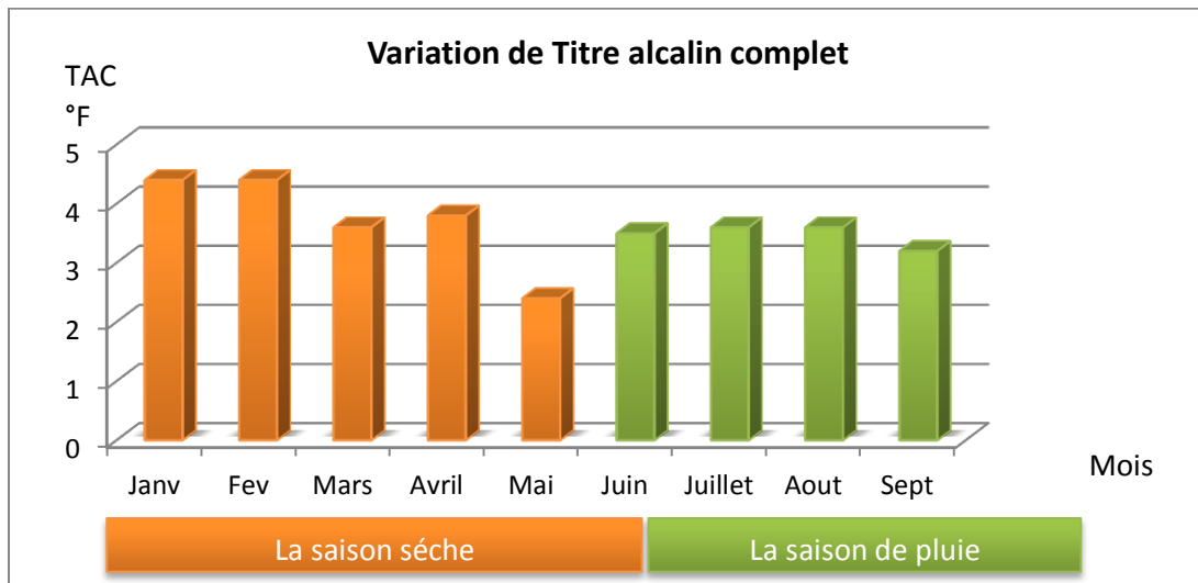
Figure 12 : Variation du titre alcalin Complet
