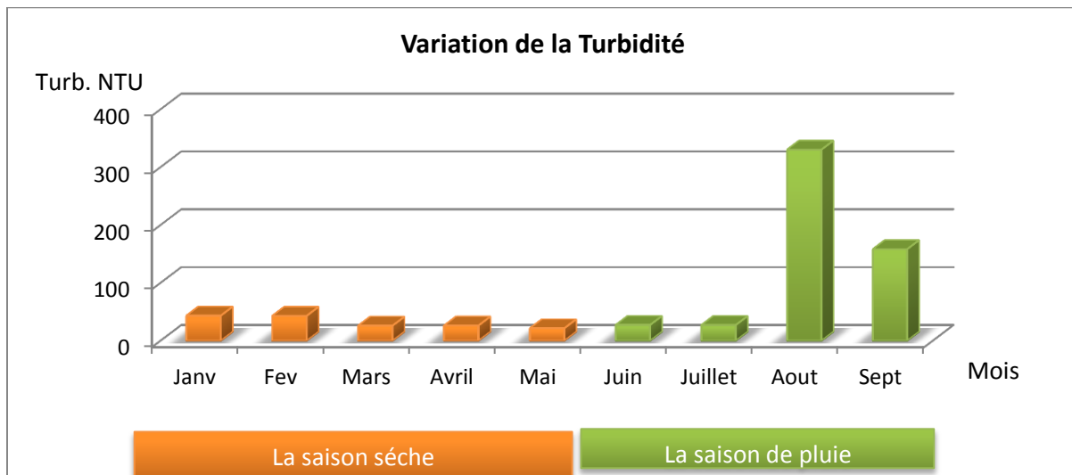
Figure 4:- Variation de la turbidité
