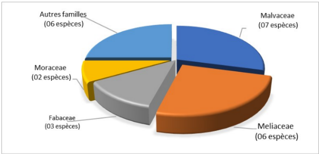
Figure 3 : Spectre de la répartition des familles dominantes des individus adultes
