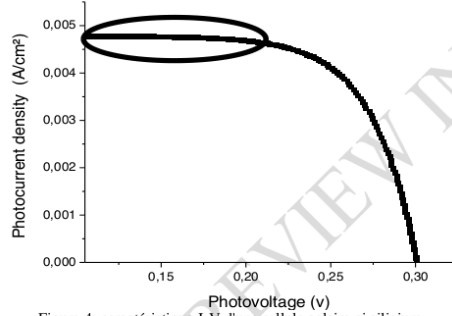
Figure 4: caractéristique J-V d'une cellule solaire au silicium
