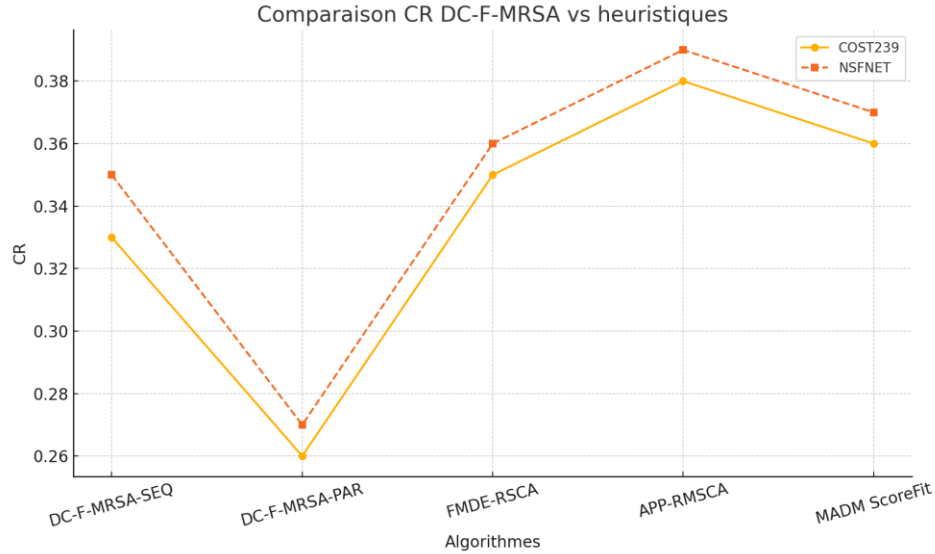
Figure-6 : DC-F-MRSA vs Heuristics
