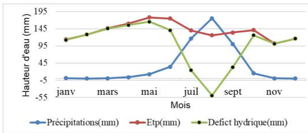
Figure 6: Representation du déficit hydrique mensuel sur la période de l'étude 1992-2023
