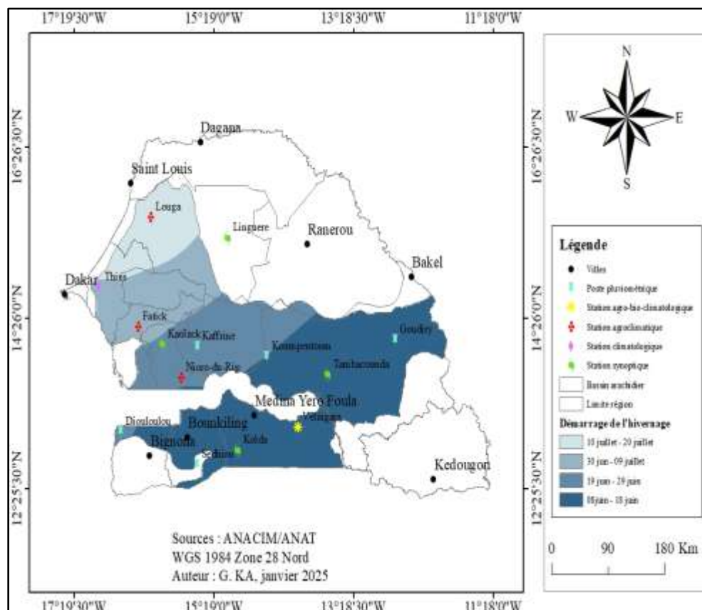
Figure 3 : Variabilité spatiale des dates de début de la saison des pluies de 1950 à 2022
