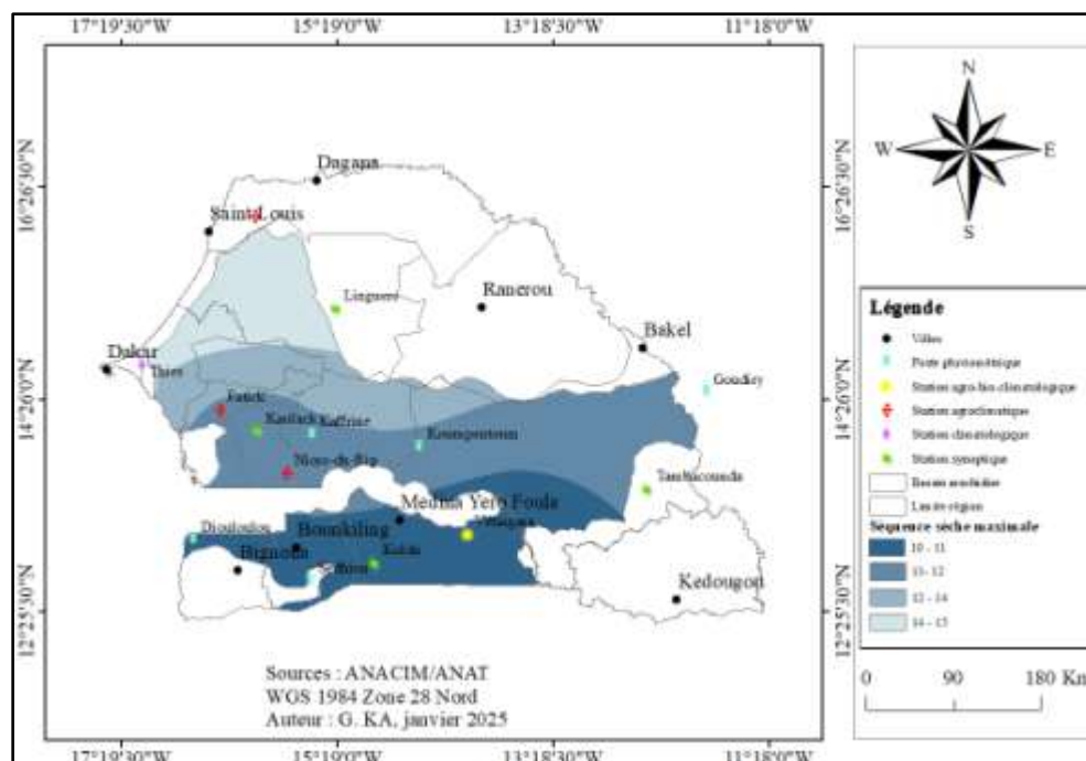
Figure 9 : Variabilité spatiale des sequences seches moyennes dans le Bassin arachidier entre 1950 et 2022
