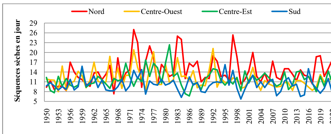
Figure 10 : Evolution interannuelle des sequences seches maximales dans le Bassin arachidier entre 1950 et 2022
