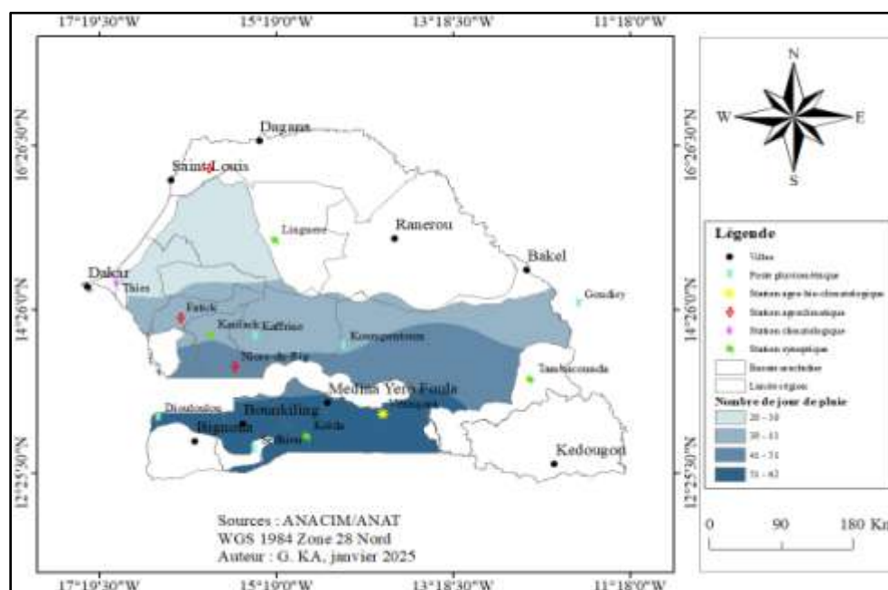
Figure 11 : Variabilite spatiale du nombre de jours de pluie dans le Bassin arachidier entre 1950 et 2022
