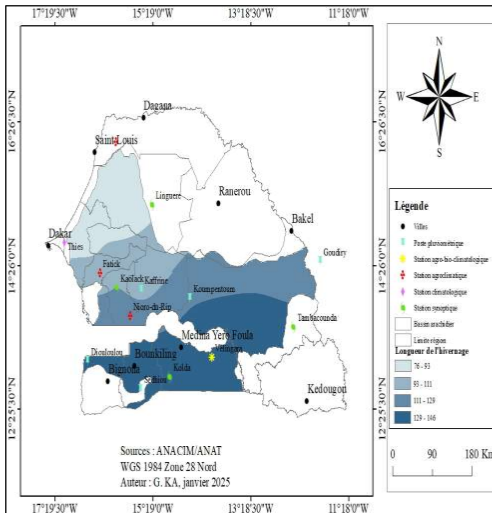
Figure 7 : Variabilité spatiale de la longueur de l'hivernage dans le Bassin arachidier entre 1950 et 2022
