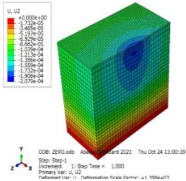
Figure 12: Champ de deflexions à la surface de la chaussée (cycle 0)
