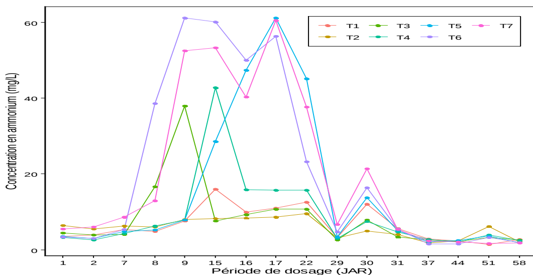
Figure 1 : Dynamique de lixiviation de l'ammonium
