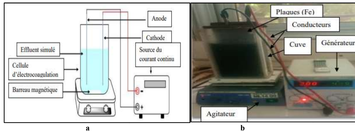
Figure 2 : a Schémas analytique du dispositif d'électrocoagulation [4].
