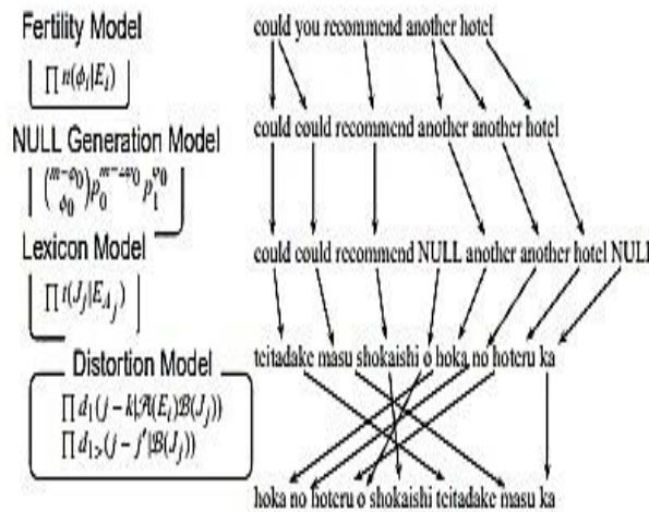
Fig 1:- Example 1.
